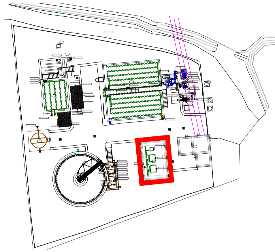
PIANTA CHIAVE - SCALA 1:500
