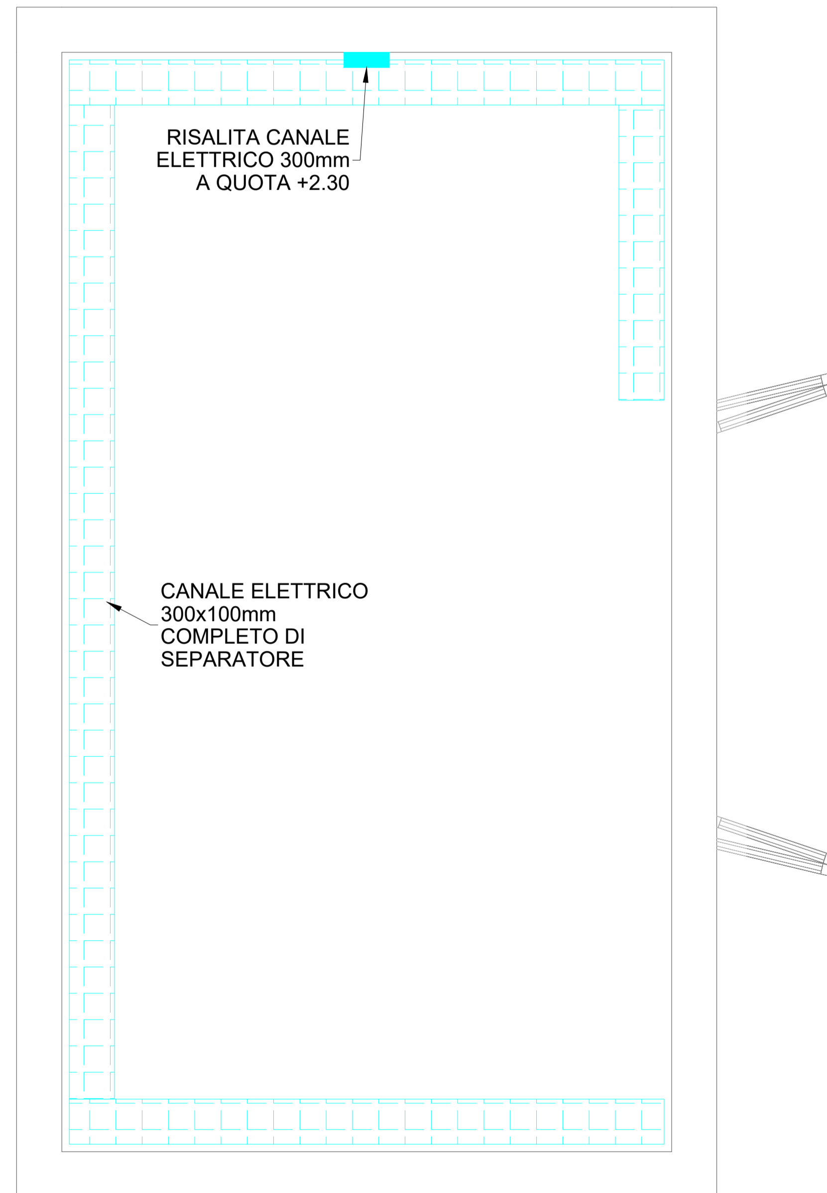
LAYOUT CANALE ELETTRICO - SCALA 1:25
