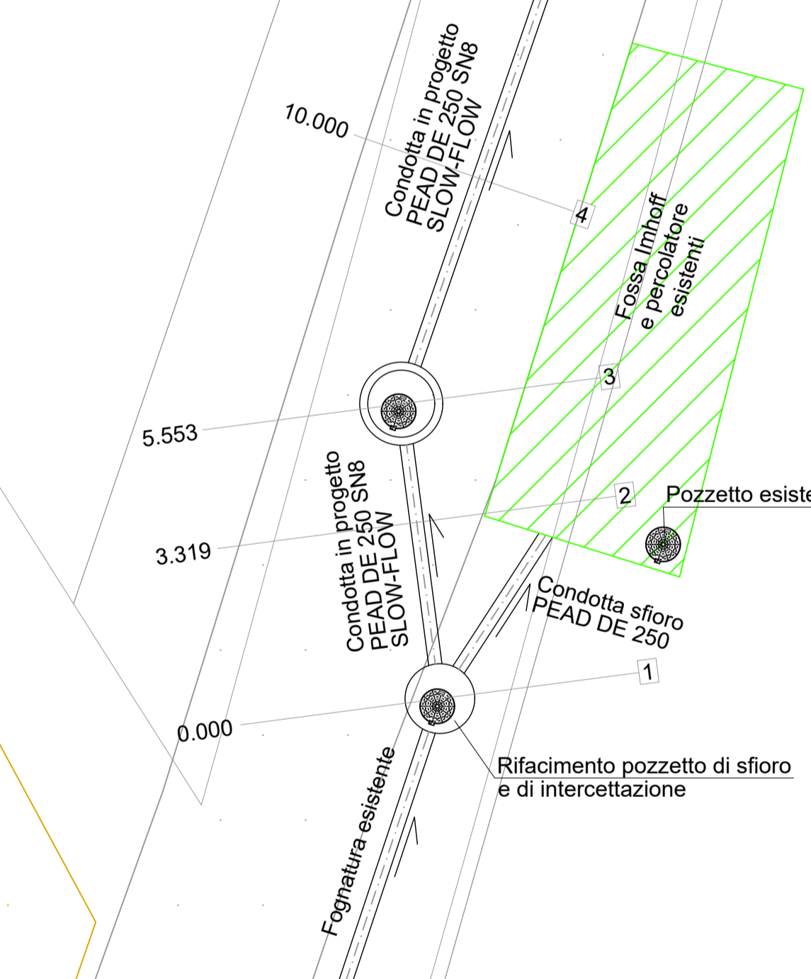
Particolare collegamenti idraulici del nuovo pozzetto di sfioro e di intercettazione Scala 1:100
