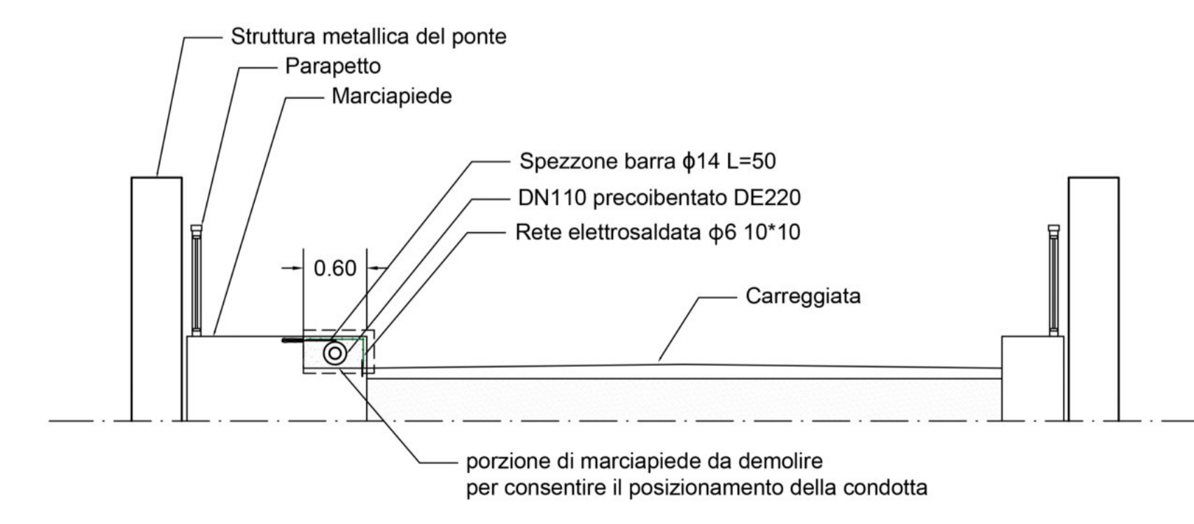
SEZIONE XX - SCALA 1:50
