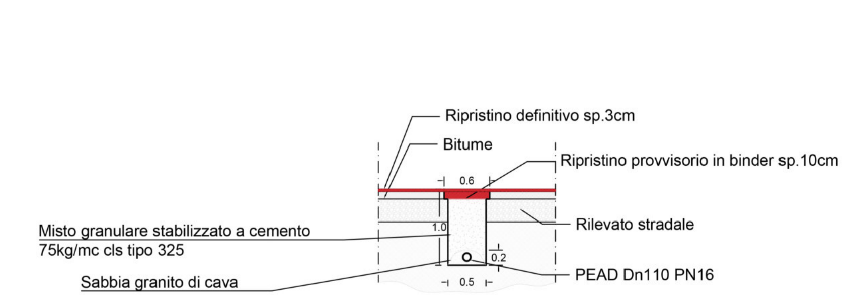
SEZIONE GENERICA SU STRADA PROVINCIALE - SCALA 1:50
