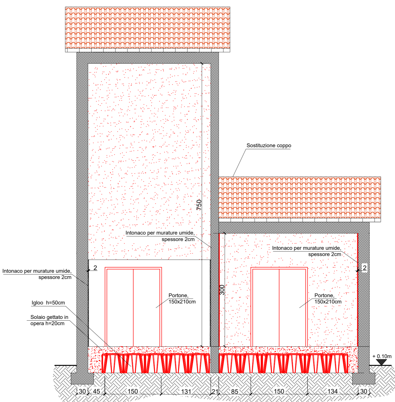
SEZIONE B-B' Scala 1:50
