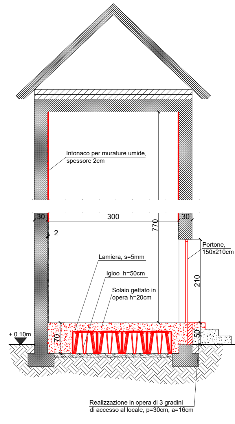
SEZIONE C-C' Scala 1:50
