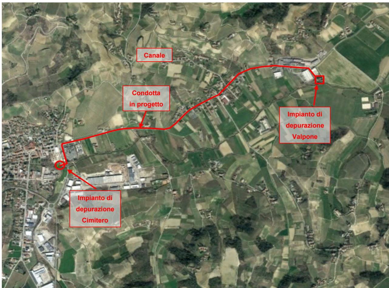
Figura 1 – Individuazione interventi
