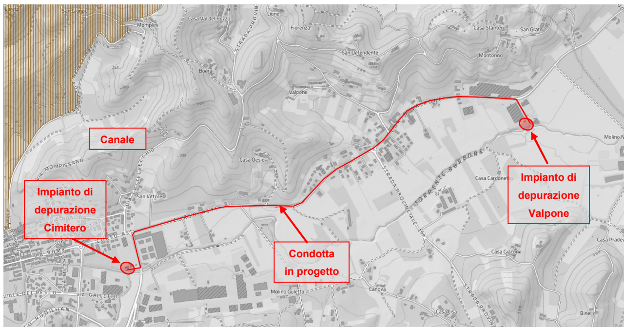
Figura 4 – Vincolo idrogeologico 5
