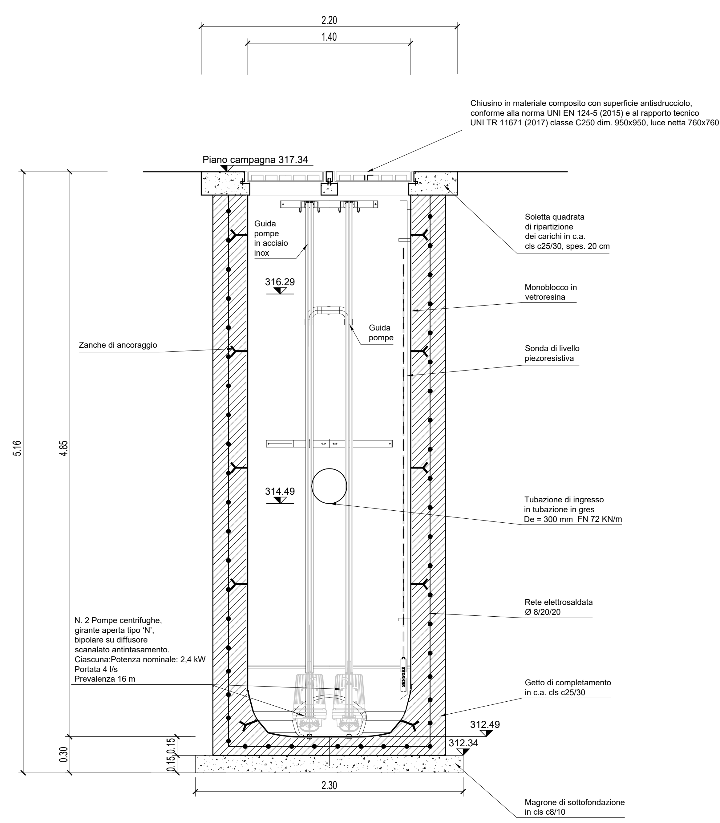
SEZIONE A - A Scala 1:20
