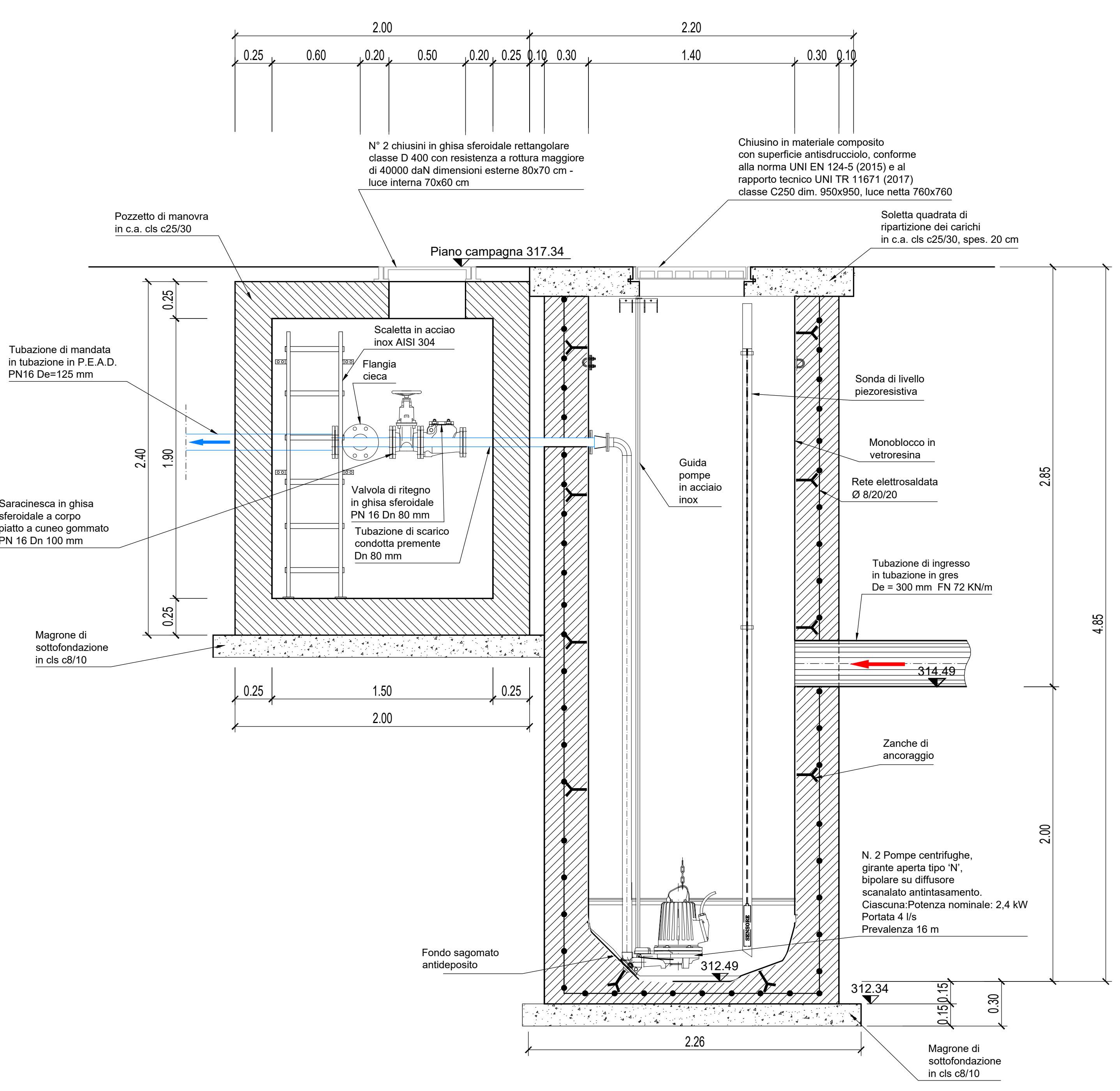
SEZIONE B - B Scala 1:20
