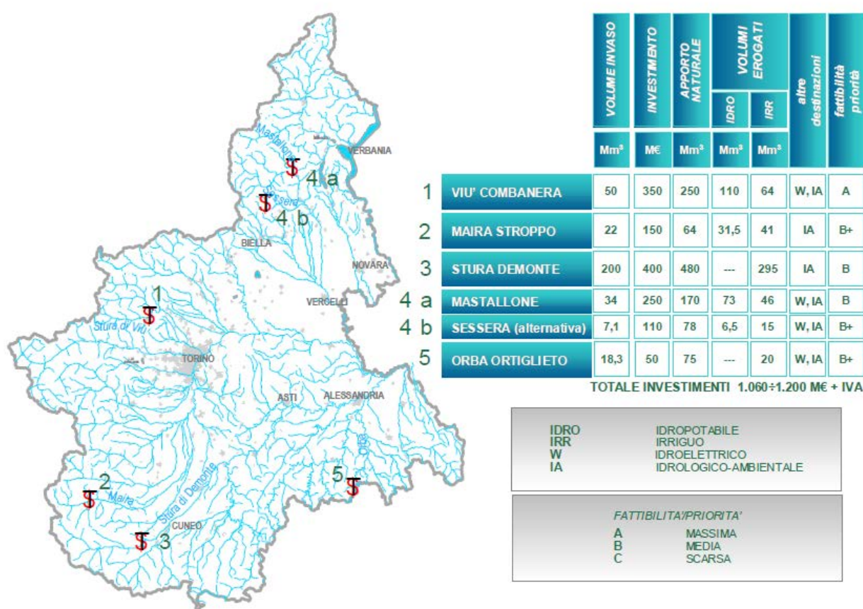
Figura 61 – Ubicazione, utilizzo, caratteristiche e priorità dei nuovi invasi a regolazione stagionale previsti nel PTA.
