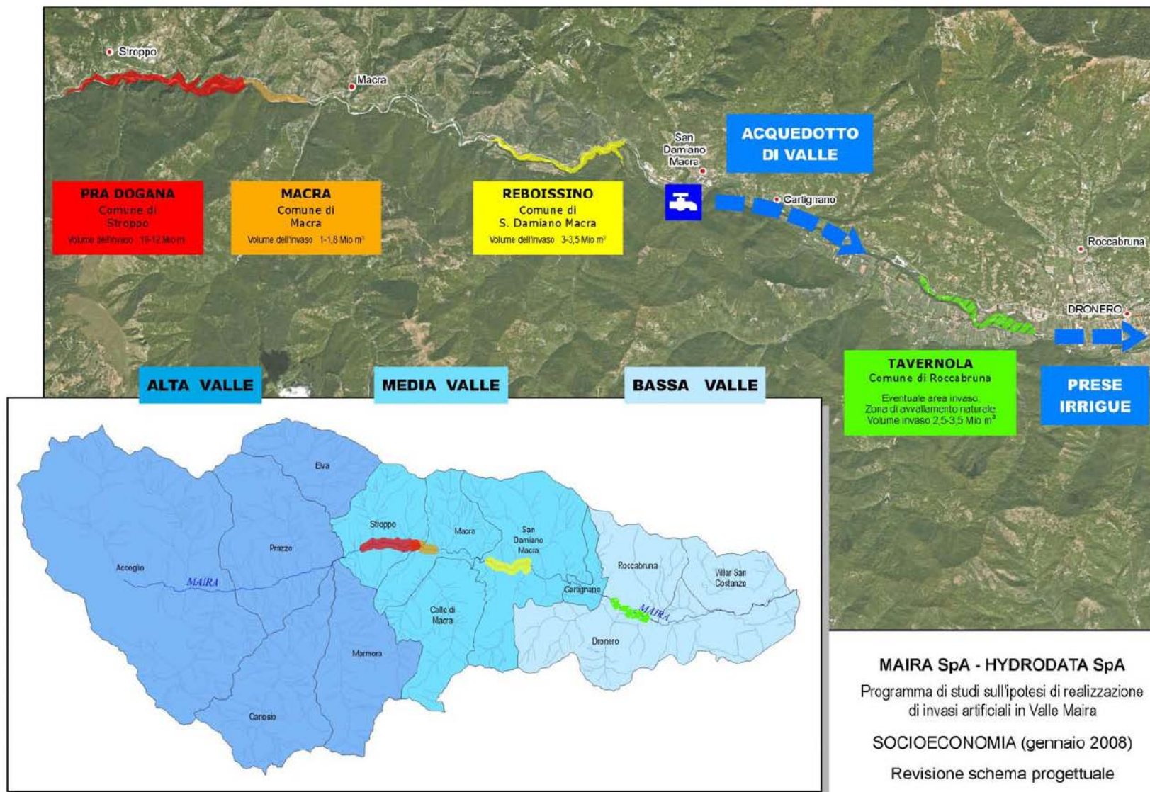
Figura 63 – Revisione dello schema progettuale relativo all'ipotesi di realizzazione di invasi artificiali in Val Maira 80 .
