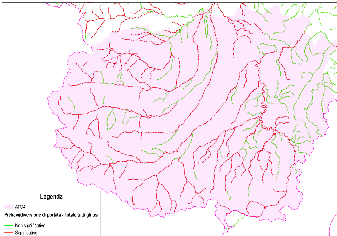
Figura 46 – Prelievo/diversione di portata: livello di pressione calcolato per tutti gli usi per i CI compresi nei territori dell'ATO4.
