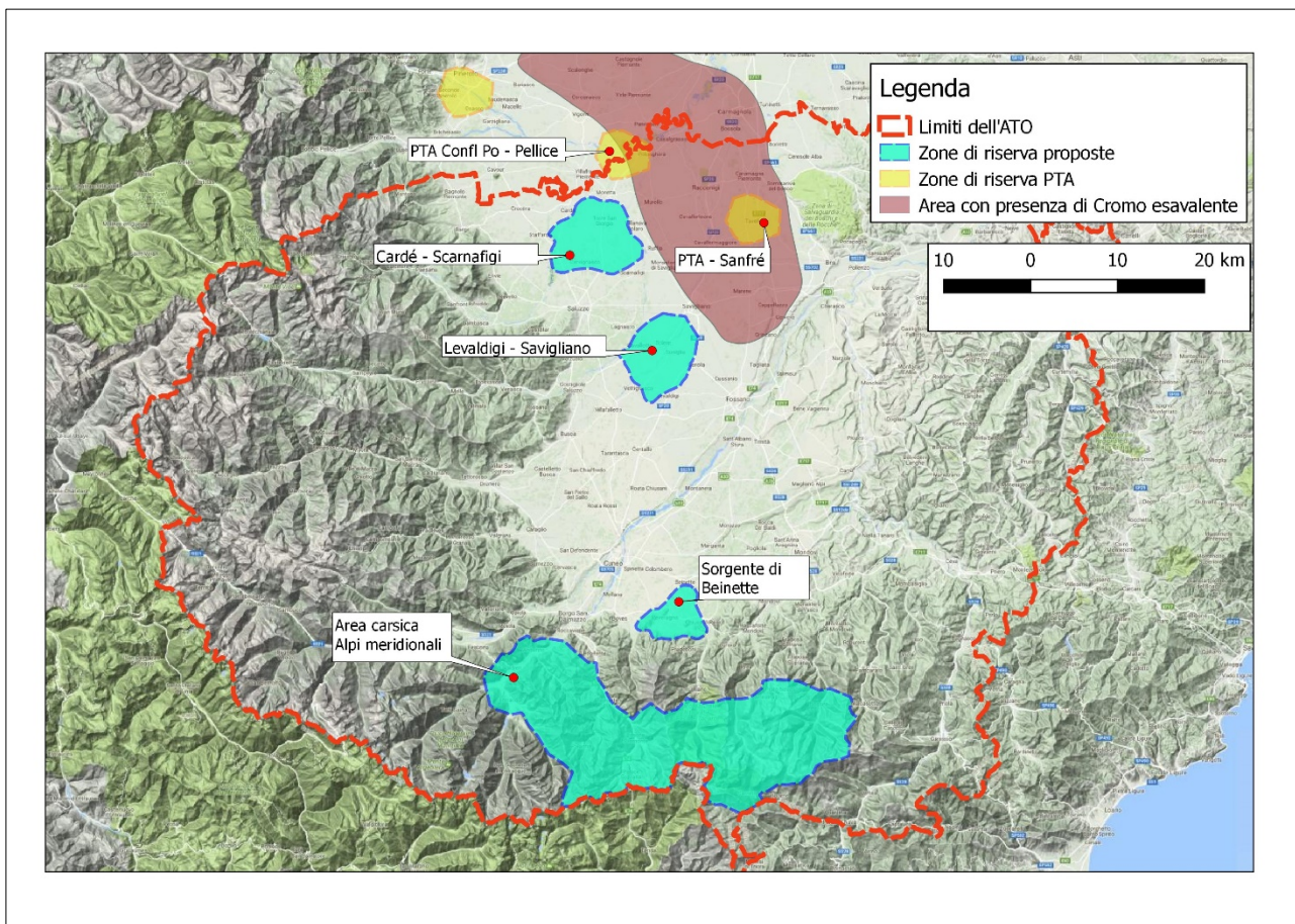
Figura 65 – Zone di riserva acque sotterranee da PTA e proposte
