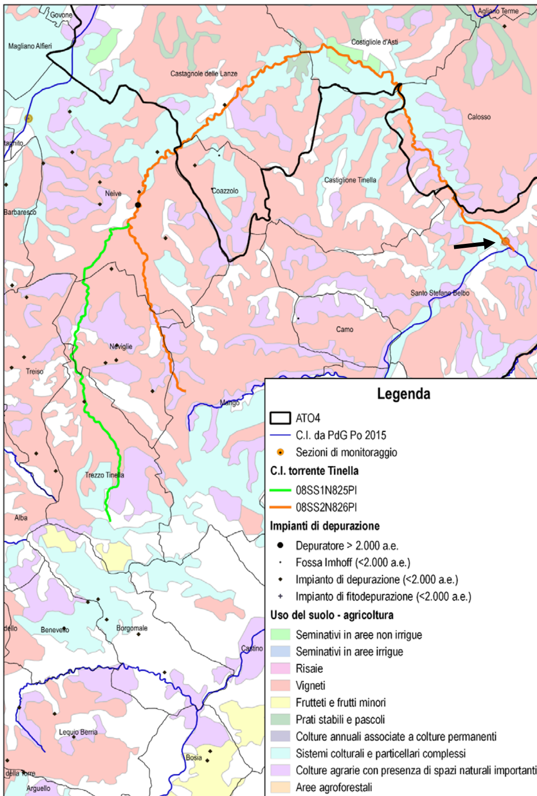
Figura 49 – Corpi idrici sul torrente Tinella nei territori dell'ATO4 ed individuazione delle sezioni di monitoraggio corrispondenti.
