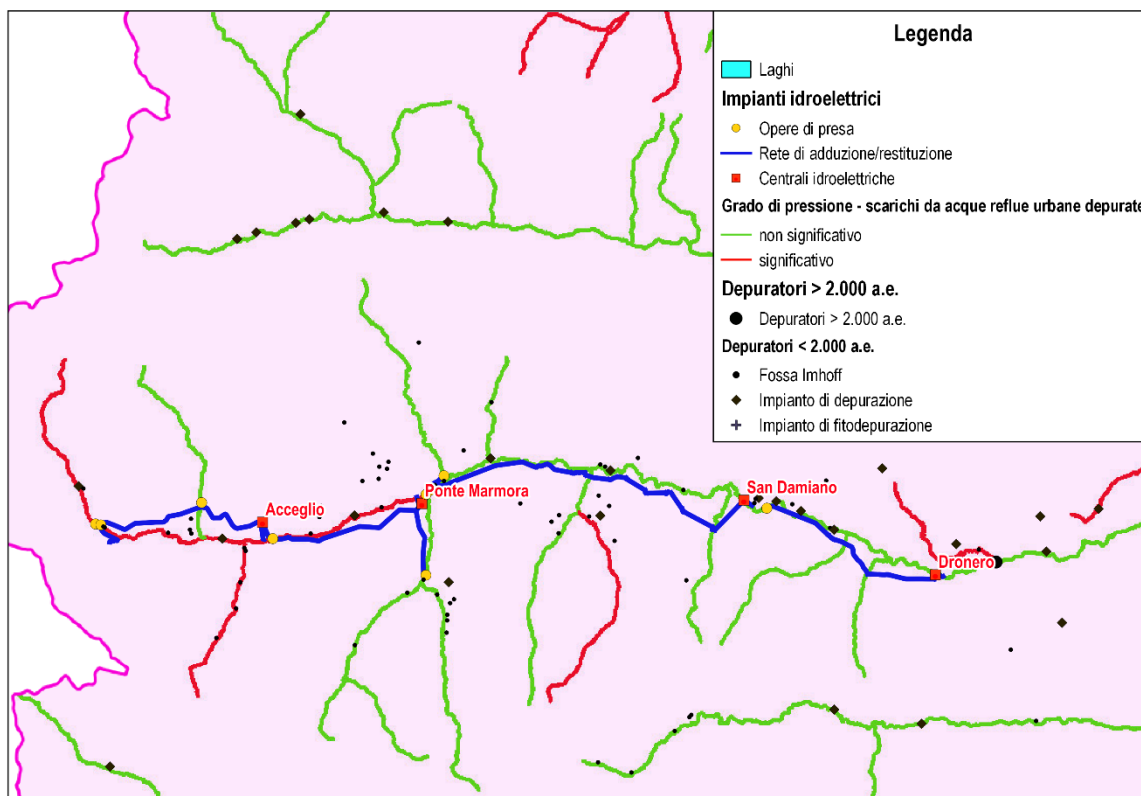
Figura 60 – Grado di pressione per scarichi da acque reflue urbane depurate, ubicazione degli impianti di depurazione esistenti e sistemi idroelettrici presenti nel tratto di interesse.
