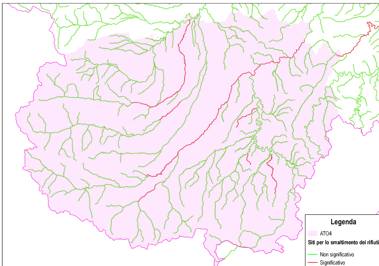
Figura 44 – Siti per lo smaltimento dei rifiuti: livello di pressione per i CI compresi nei territori dell'ATO4.
