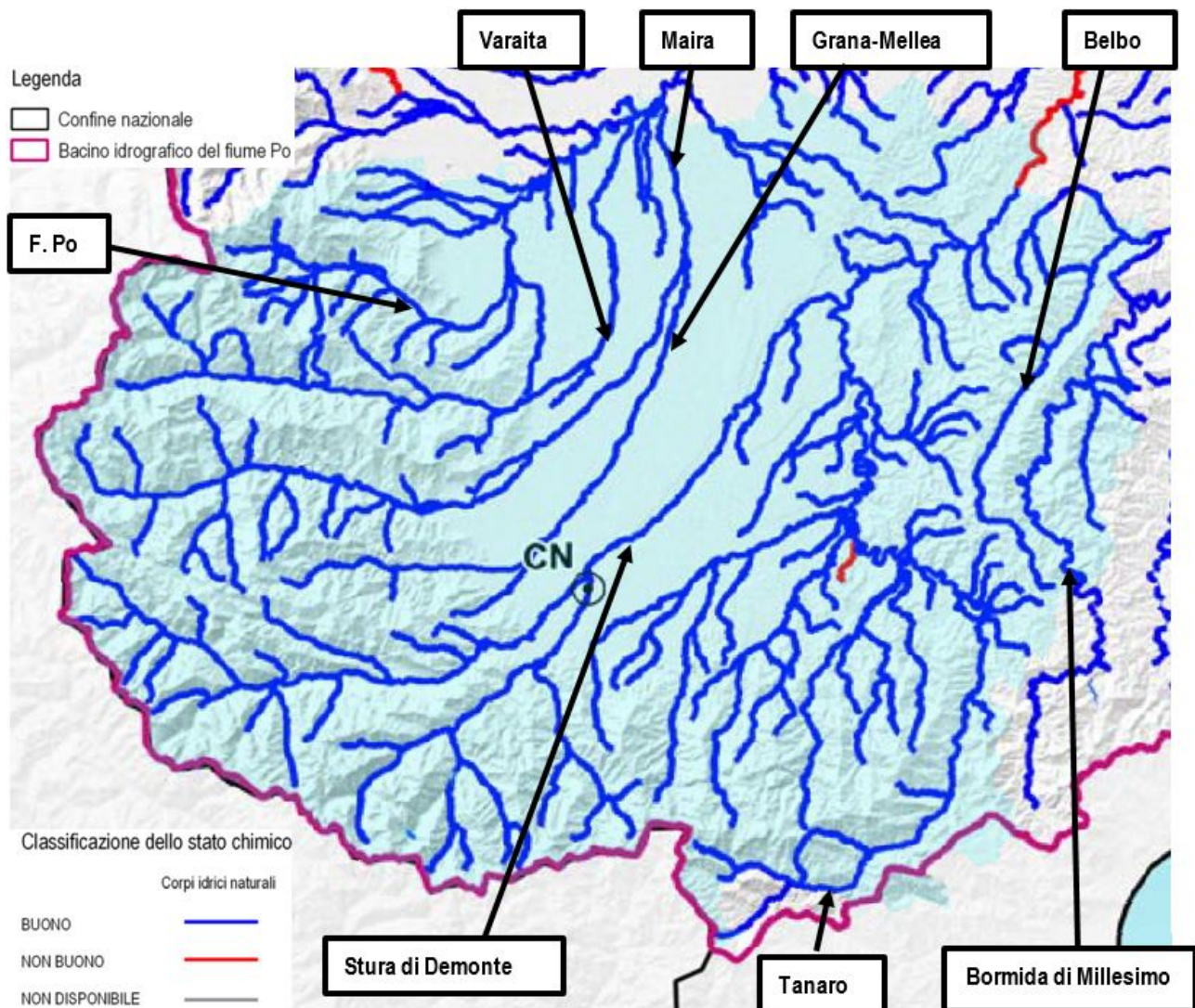
Figura 12 - Classificazione dello stato chimico dei C.I. (fonte AdB Po) con evidenziati i territori dell'ATO 4.
