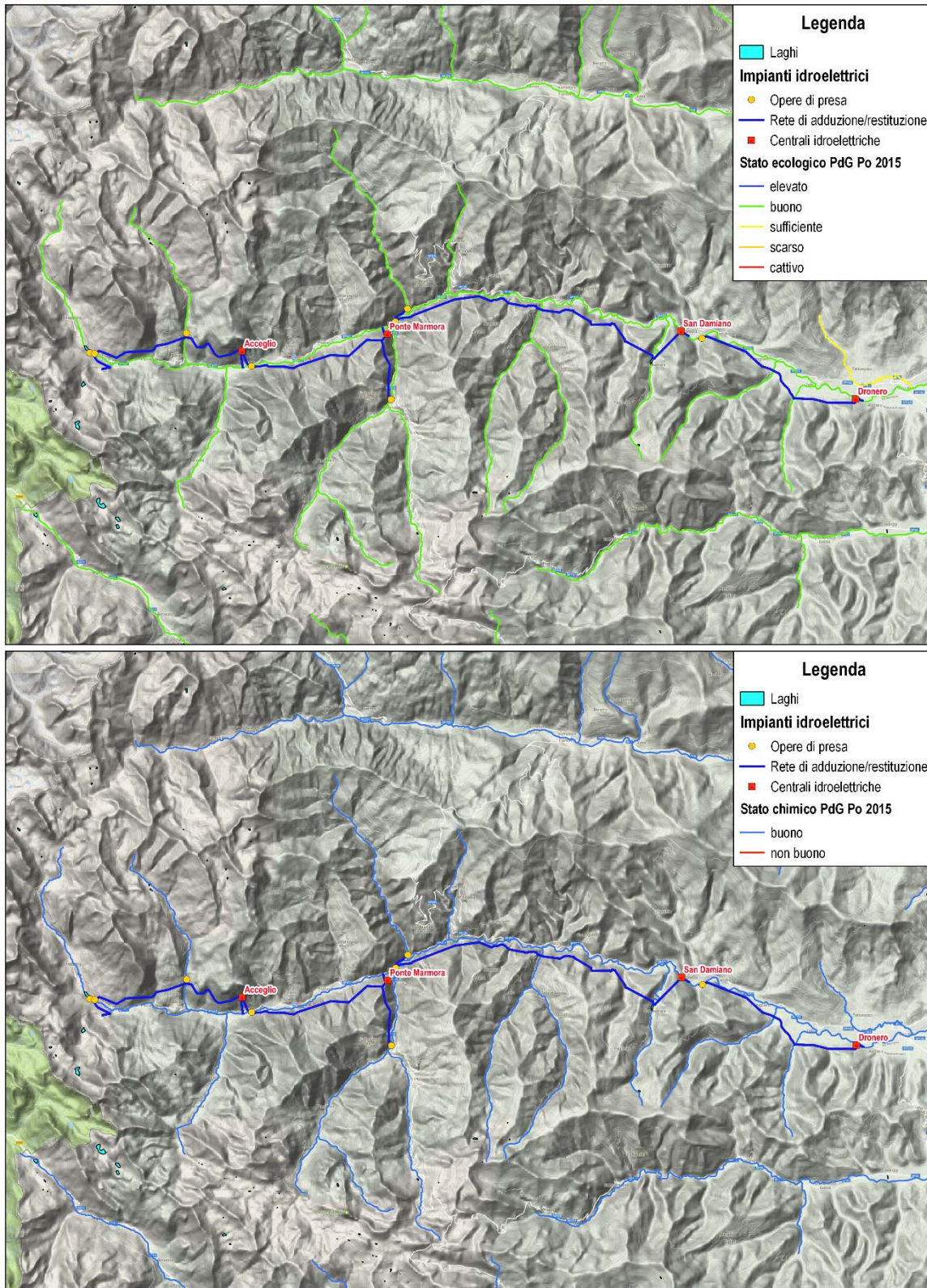
Figura 59 – Stato ecologico (sopra) e chimico (sotto) dei C.I. interessati dalle derivazioni dei sistemi idroelettrici presenti sul torrente Maira a monte di Dronero.
