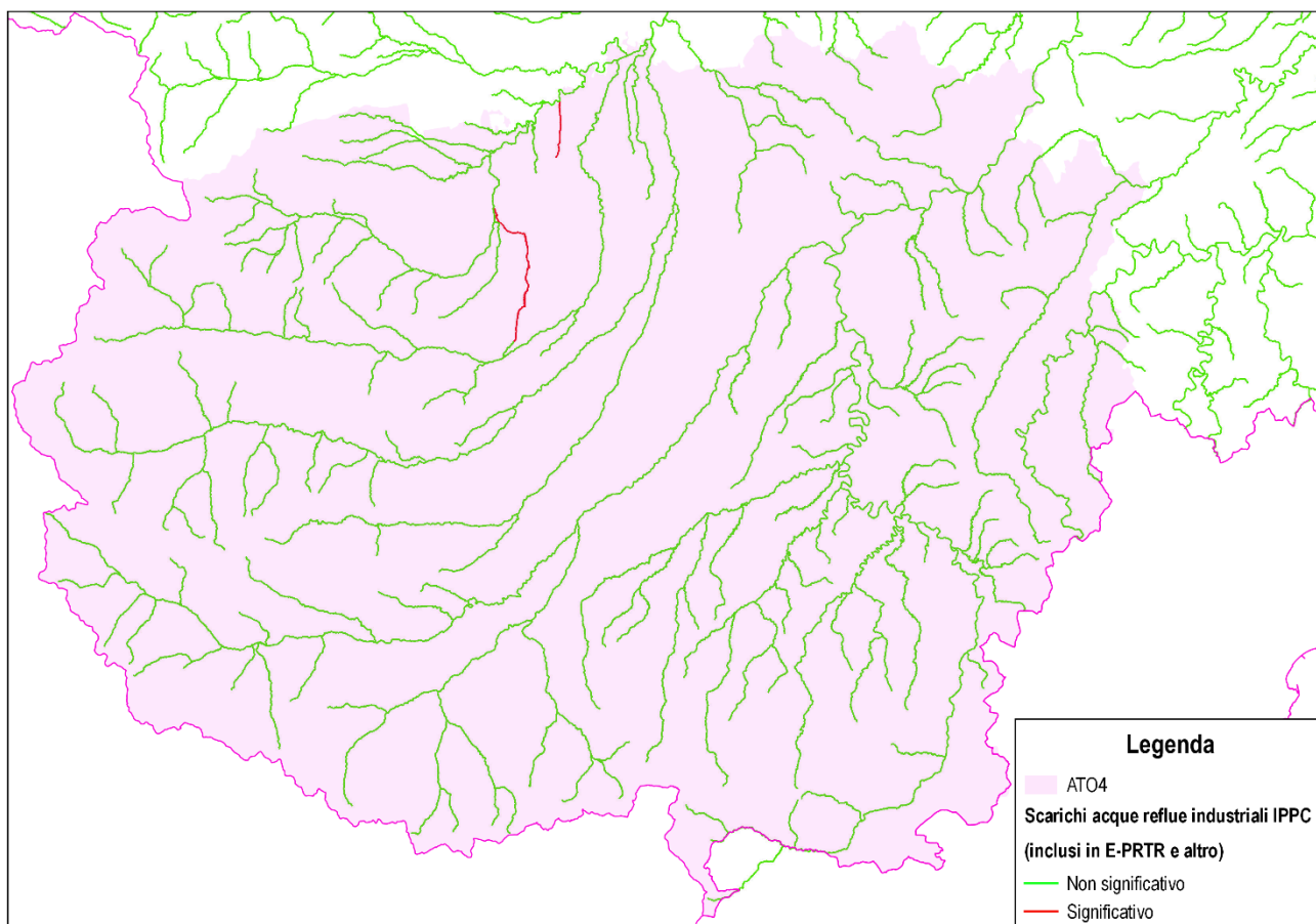
Figura 41 – Scarico da acque reflue industriali IPPC: livello di pressione per i CI compresi nei territori dell'ATO4.
