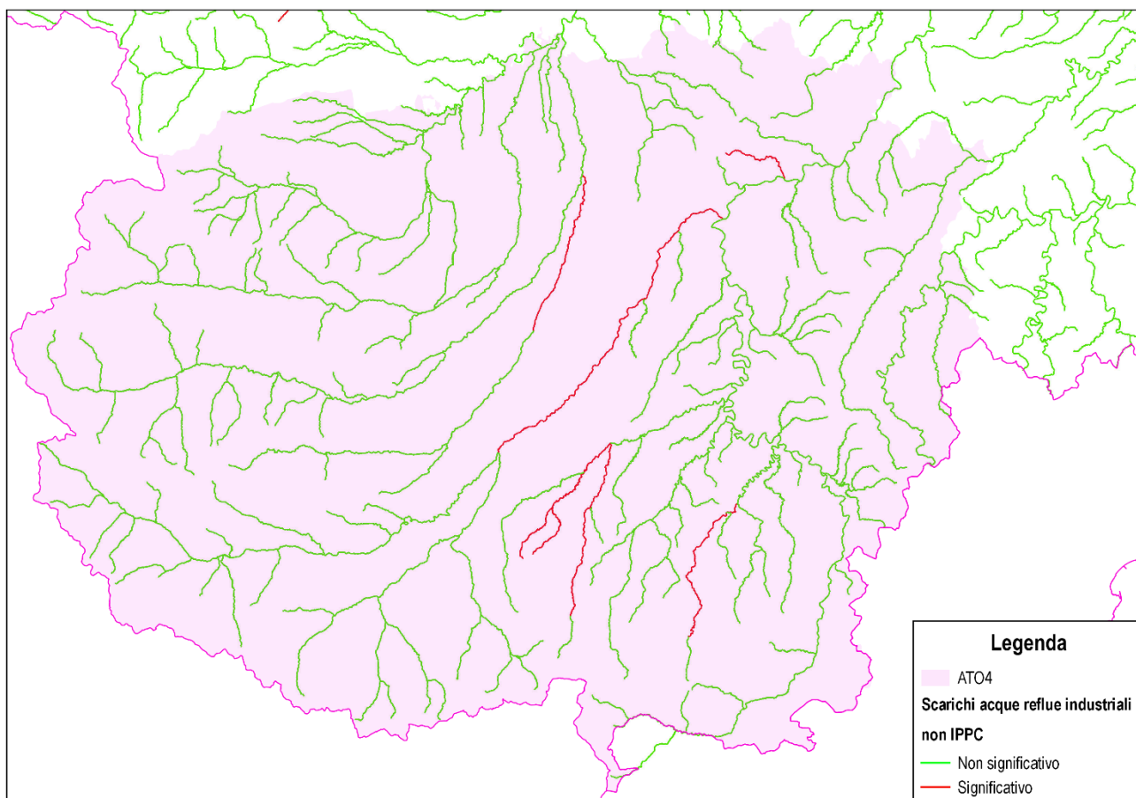
Figura 42 – Scarico da acque reflue industriali non IPPC: livello di pressione per i CI compresi nei territori dell'ATO4.
