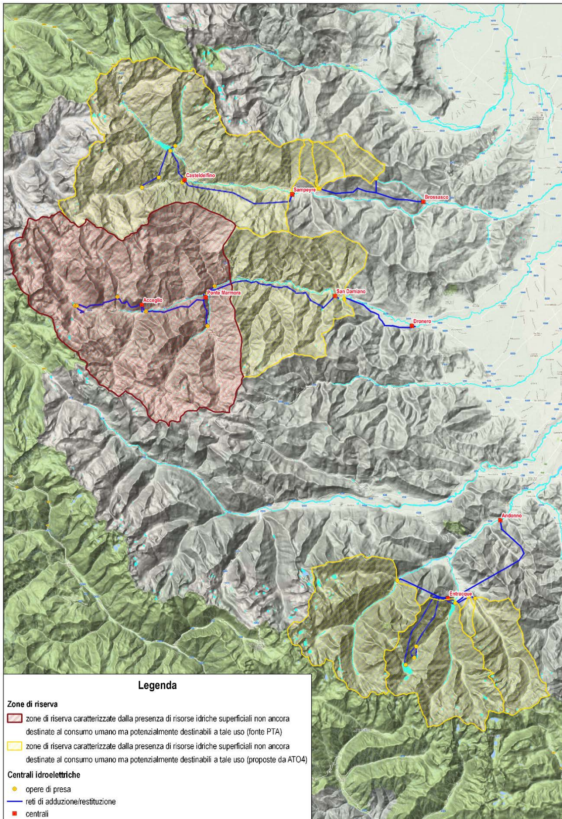
Figura 64 – Zone di riserva delle acque superficiali destinate al consumo umano.
