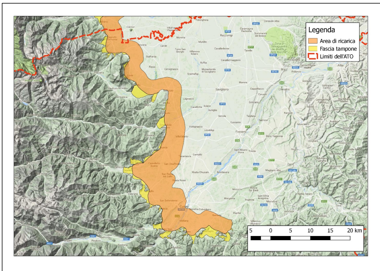
Figura 53 – Aree di ricarica e fasce tampone nel territorio dell'ATO
