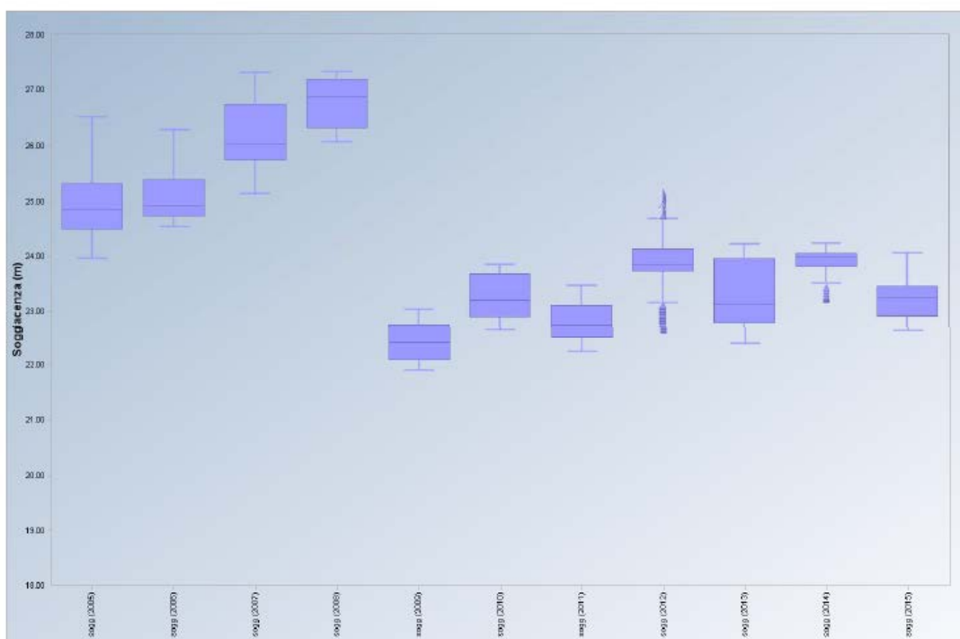
Figura 32 - Andamento della soggiacenza in funzione delle piogge – in alto – e sotto forma di box plot in basso (la scatola rappresenta in valori giornalieri compresi tra il 25 e 75 percentile mentre la riga in essi contenuti e la mediana; gli altri simboli riproducono l'escursione massima) alla stazione piezometrica ARPA di Tarantascai
