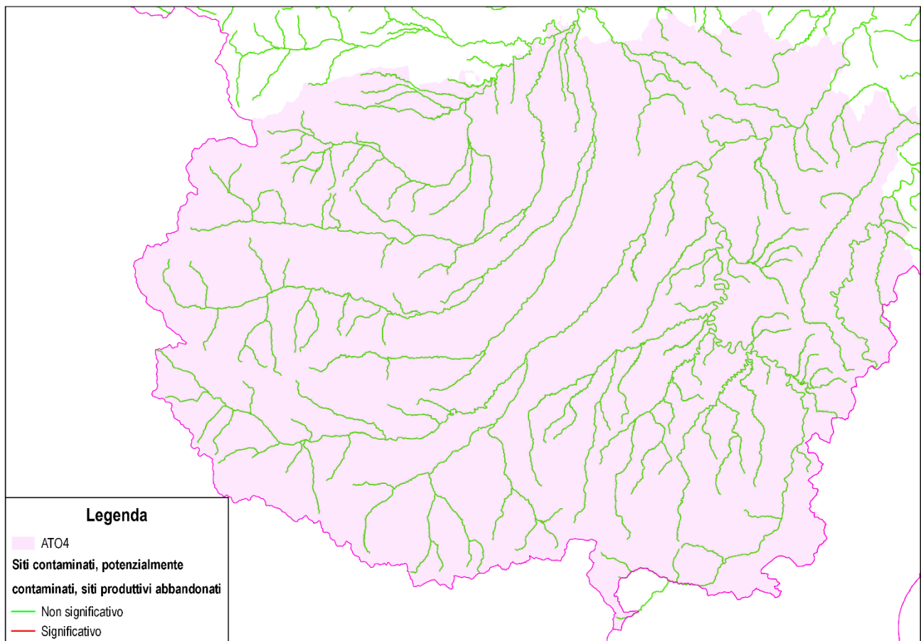
Figura 43 – Siti contaminati: livello di pressione per i CI compresi nei territori dell'ATO4.
