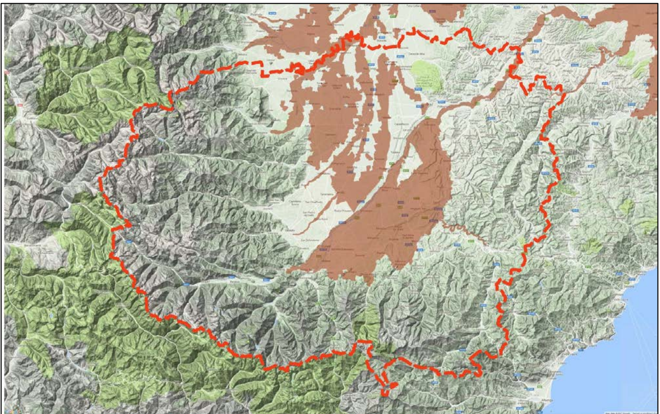
Figura 54 – Zone vulnerabili ai nitrati (in marrone = ZNV + Fascia A e B del PAI).
