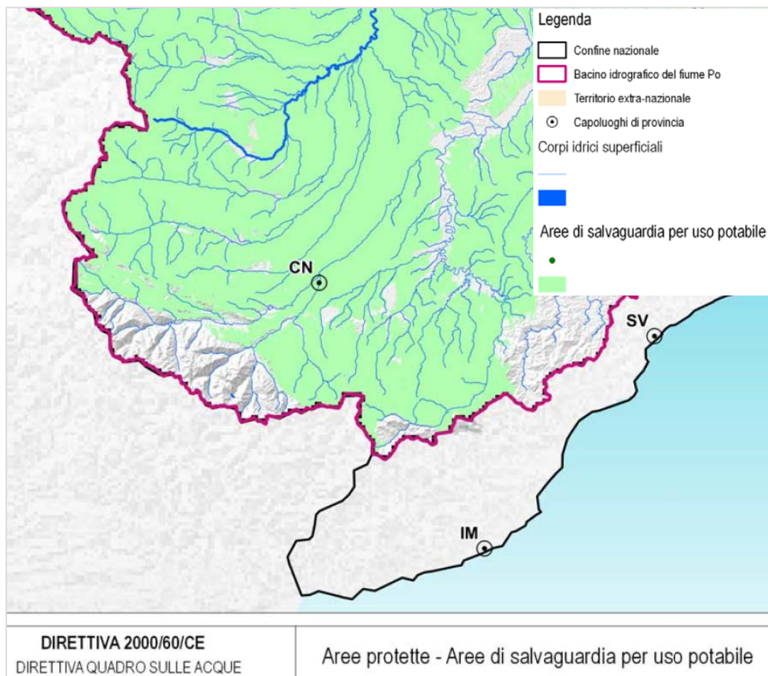
Figura 17 – Estratto dalla tavola 3.1 dell'Allegato 12.1 all'Elaborato 12 del Piano di Gestione del distretto idrografico del fiume Po (versione marzo 2016).
