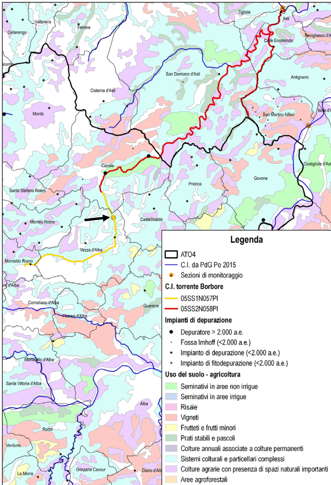
Figura 50 – Corpi idrici sul torrente Borbore nei territori dell’ATO4 ed individuazione delle sezioni di monitoraggio corrispondenti.
