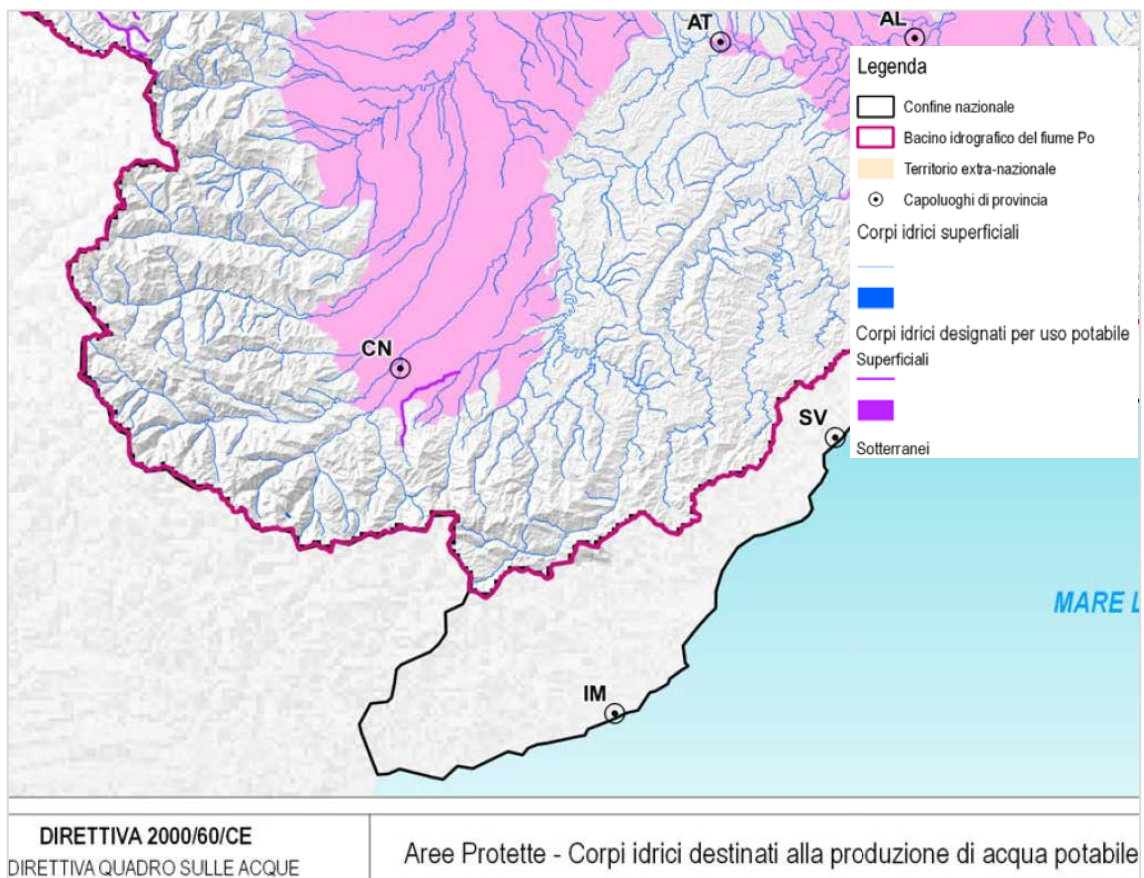
Figura 16 – Estratto dalla tavola 3.2 dell’Allegato 12.1 all’Elaborato 12 del Piano di Gestione del distretto idrografico del fiume Po (versione marzo 2016).
