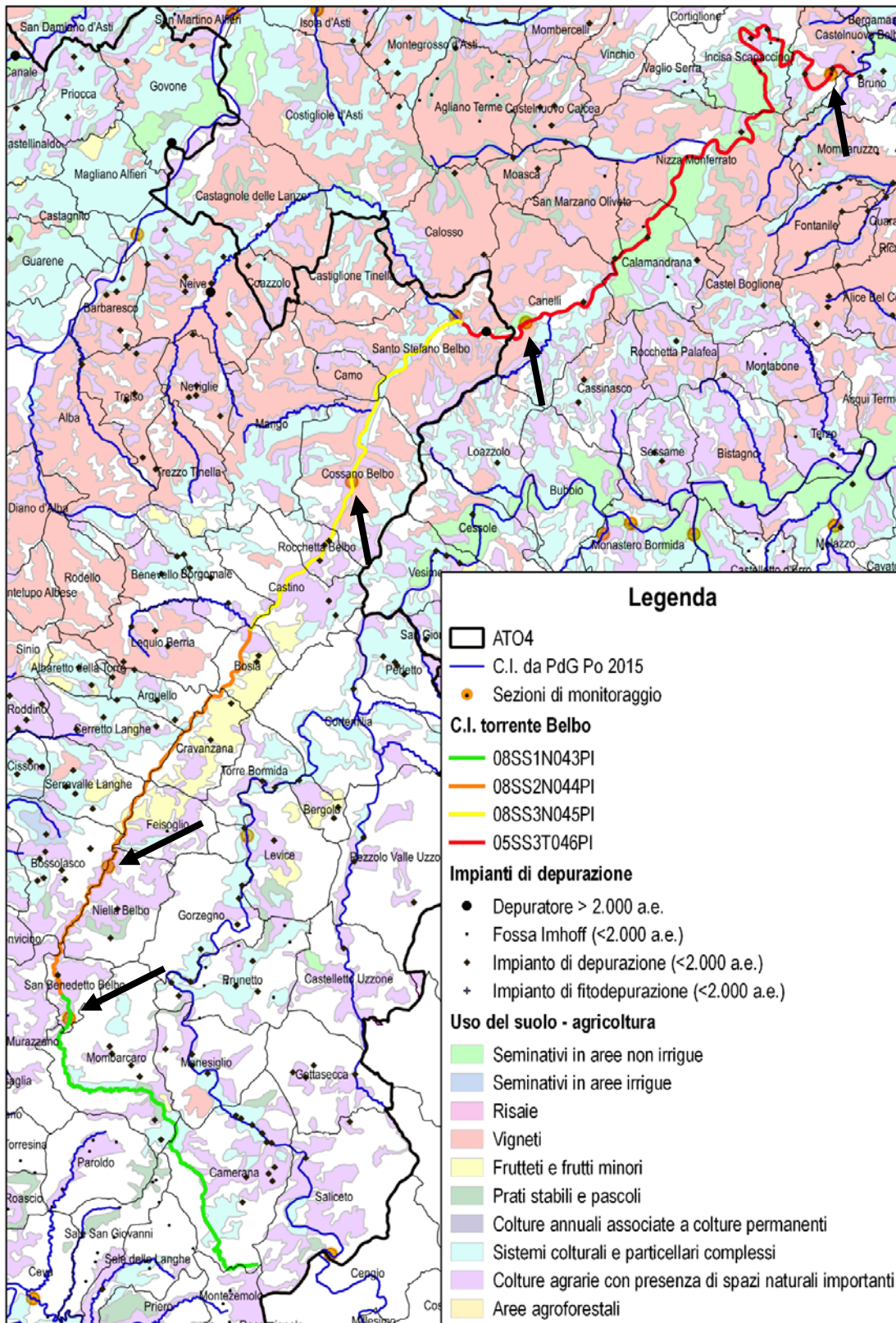
Figura 48 – Corpi idrici sul torrente Belbo nei territori dell’ATO4 ed individuazione delle sezioni di monitoraggio corrispondenti.
