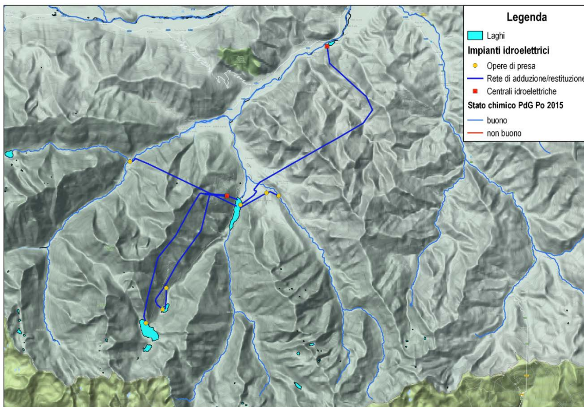
Figura 58 – Stato ecologico (sopra) e chimico (sotto) dei C.I. interessati dalle derivazioni degli impianti ENEL sull'alto bacino del torrente Gesso.
