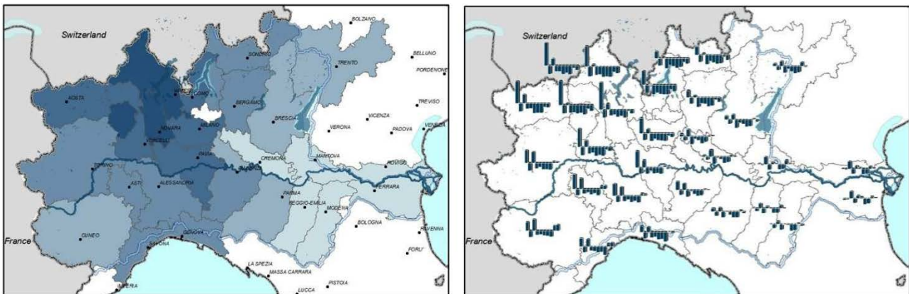
Figura 39 - Precipitazioni nel bacino del Po: (sinistra) precipitazione annua media (2000-2009) per Provincia; (destra) istogramma della variazione di precipitazione annuale negli anni 2000-2010 rispetto alla precipitazione annuale media nel periodo (1971-2000) per Provincia 39 .
