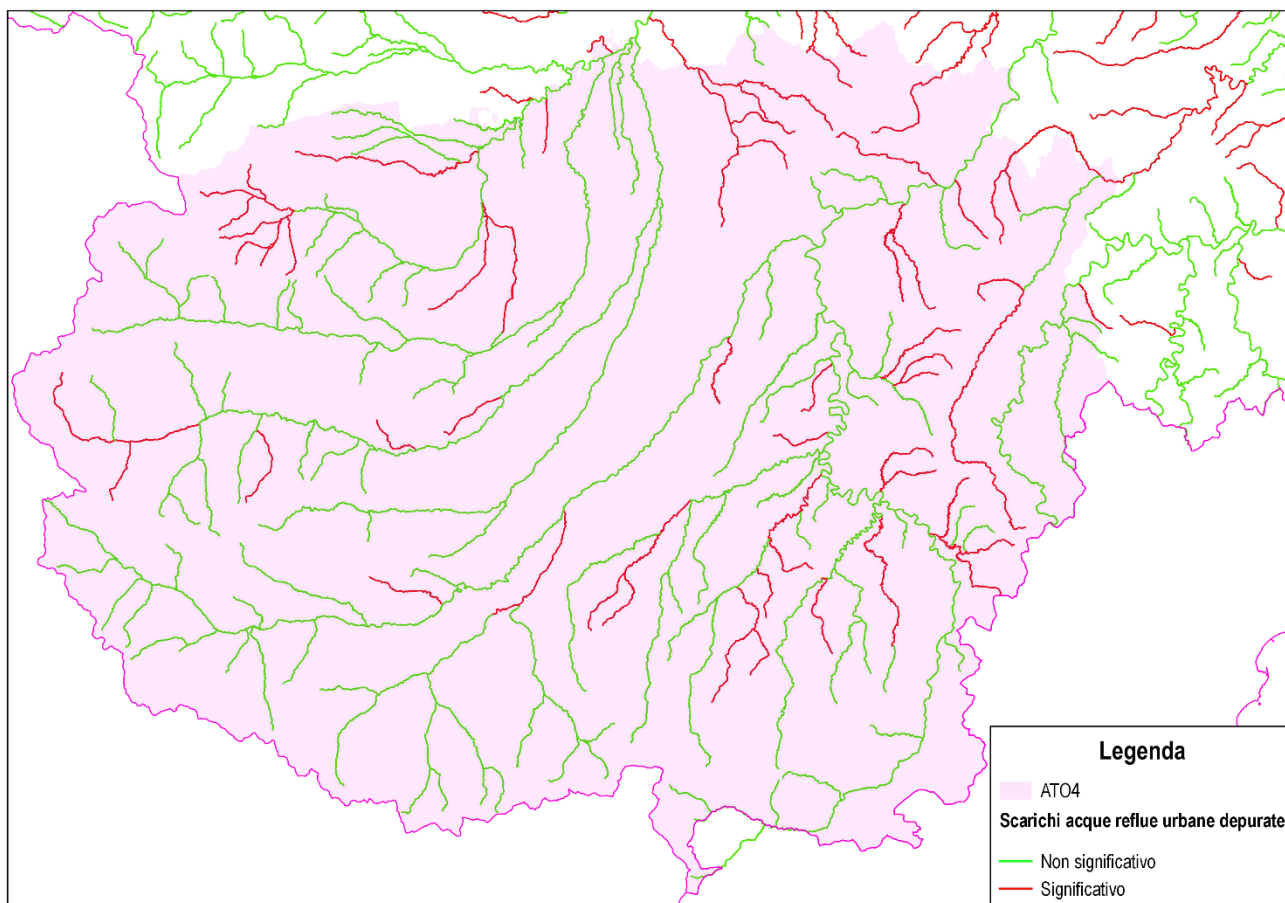
Figura 40 – Scarico da acque reflue urbane depurate: livello di pressione per i CI compresi nei territori dell'ATO4.
