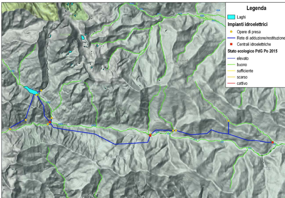
Figura 56 – Stato ecologico dei C.I. interessati dalle derivazioni degli impianti ENEL a monte di Brossasco sul torrente Varaita.
