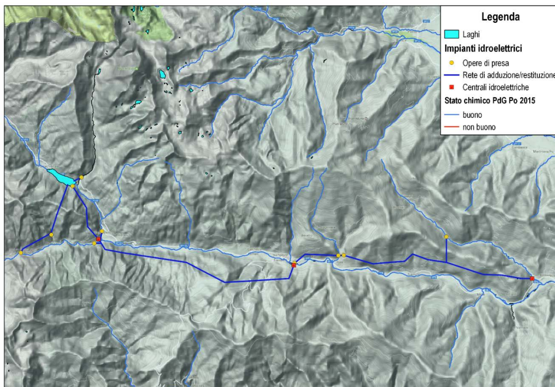
Figura 57 – Stato chimico dei C.I. interessati dalle derivazioni degli impianti ENEL a monte di Brossasco sul torrente Varaita.
