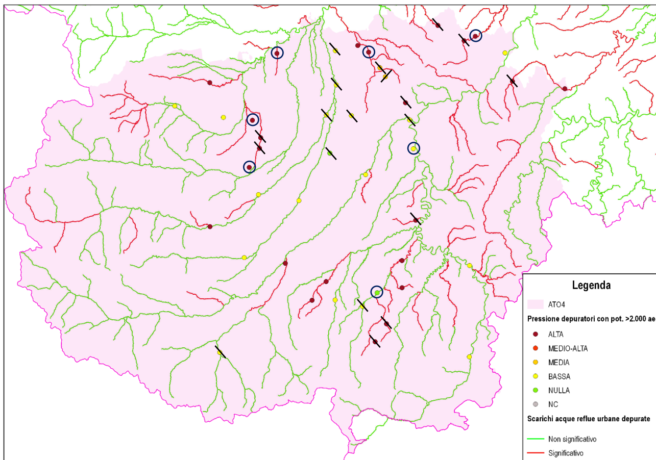
Figura 47 – Scarico da acque reflue urbane depurate: livello di pressione per i CI compresi nei territori dell'ATO4 a confronto con l'ubicazione degli impianti con potenzialità superiore a 2.000 ae. classificati in funzione del grado di pressione definito da ARPA. Il cerchio blu indica i depuratori di cui nel Pdl è previsto il potenziamento; la barra nera quelli di cui è prevista l'eliminazione.
