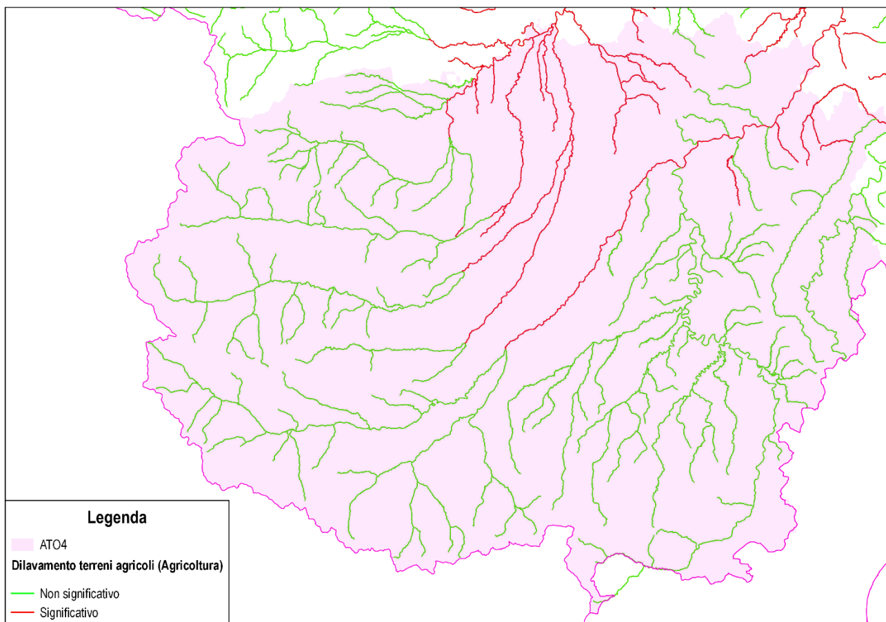
Figura 45 – Dilavamento dei terreni agricoli: livello di pressione per i CI compresi nei territori dell'ATO4.
