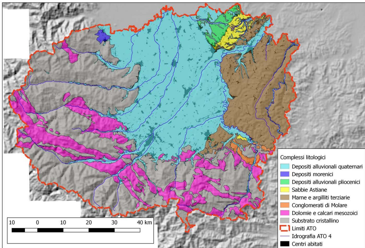
Figura 2 - Schema litologico del territorio dell'ATO4.
