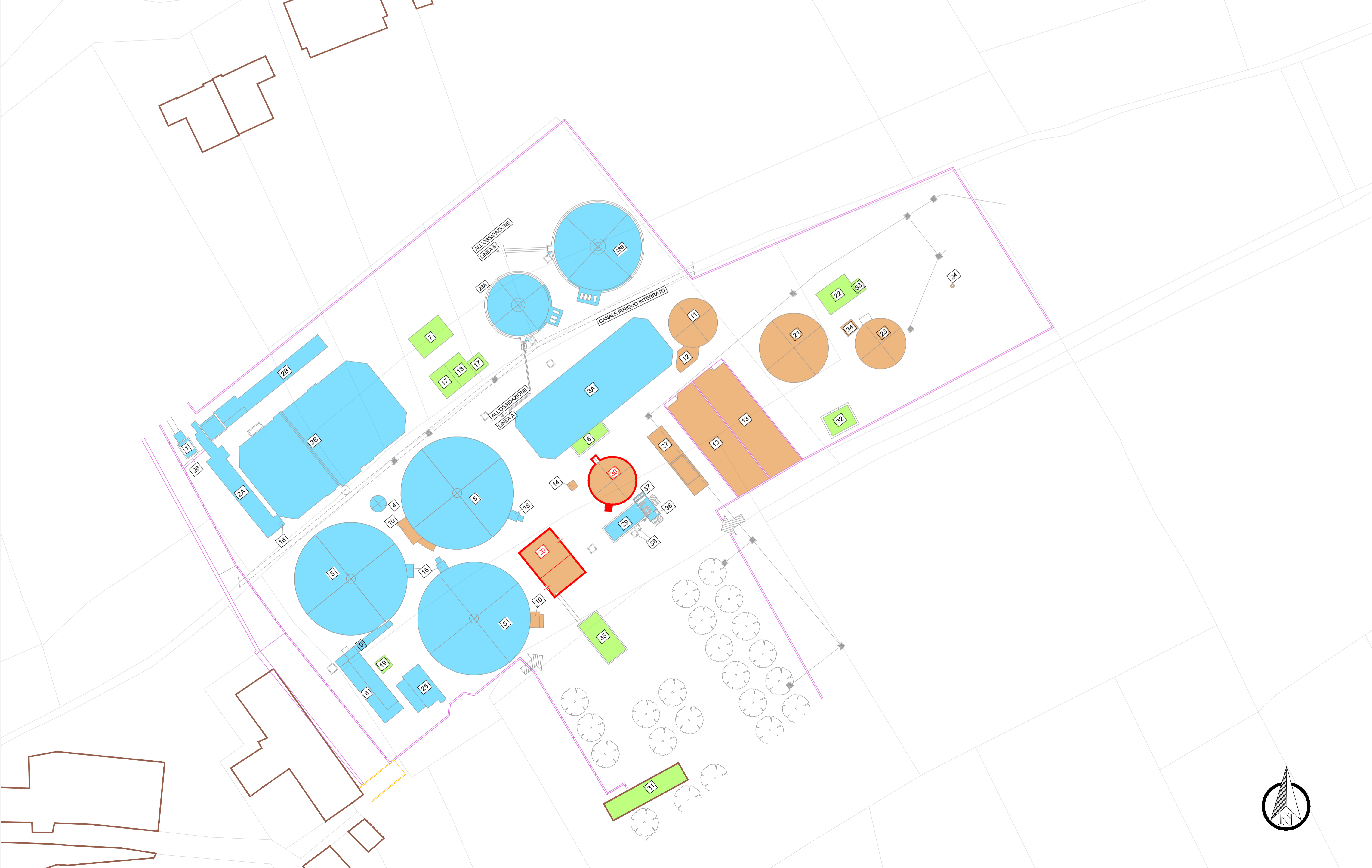
PLANIMETRIA : IMPIANTO DI DEPURAZIONE IN LOCALITA' "LA BASSA" BRA SCALA 1:500
