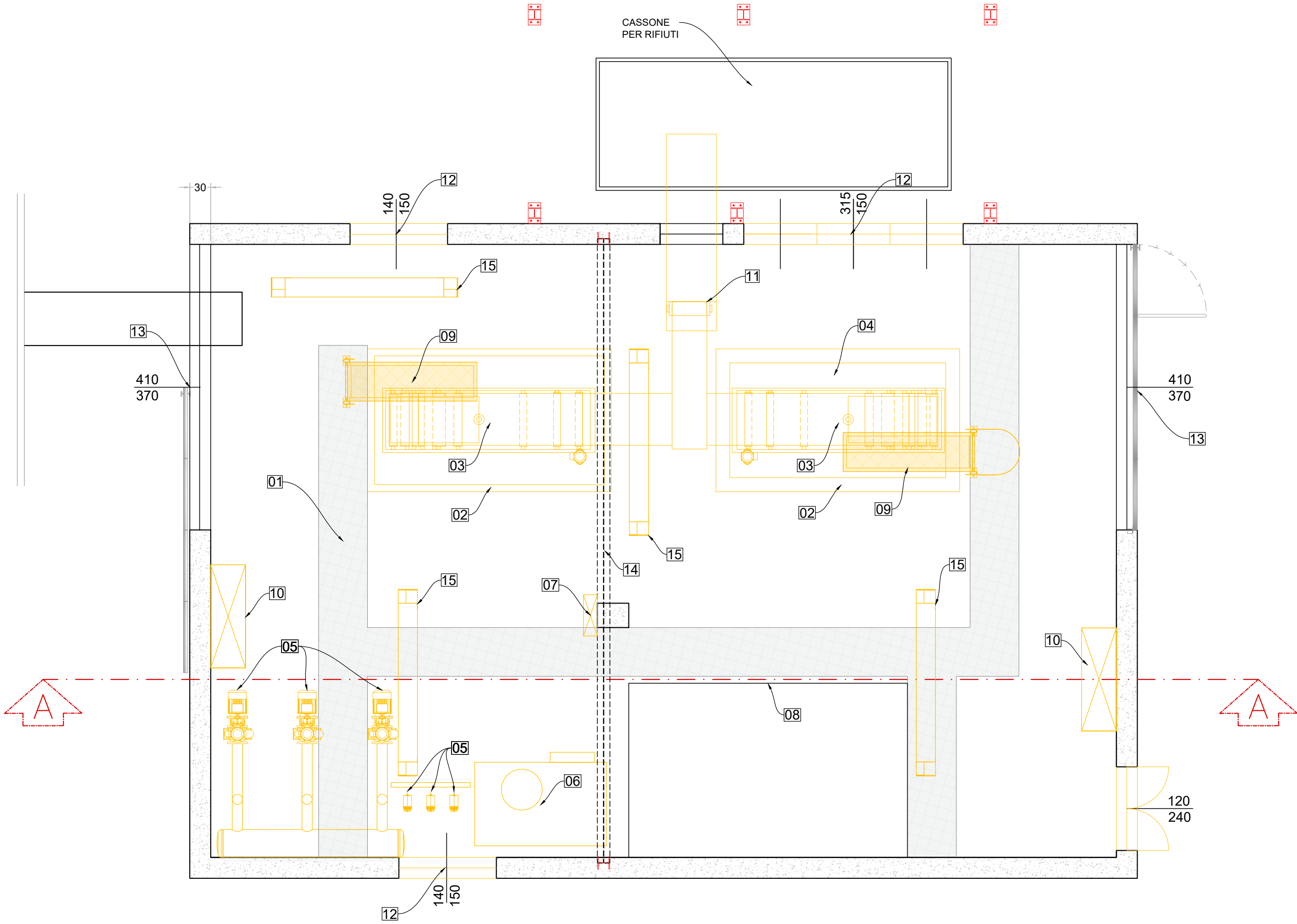
PIANTA LOCALE DISIDRATAZIONE FANGHI - STATO DI FATTO SCALA - 1:50
