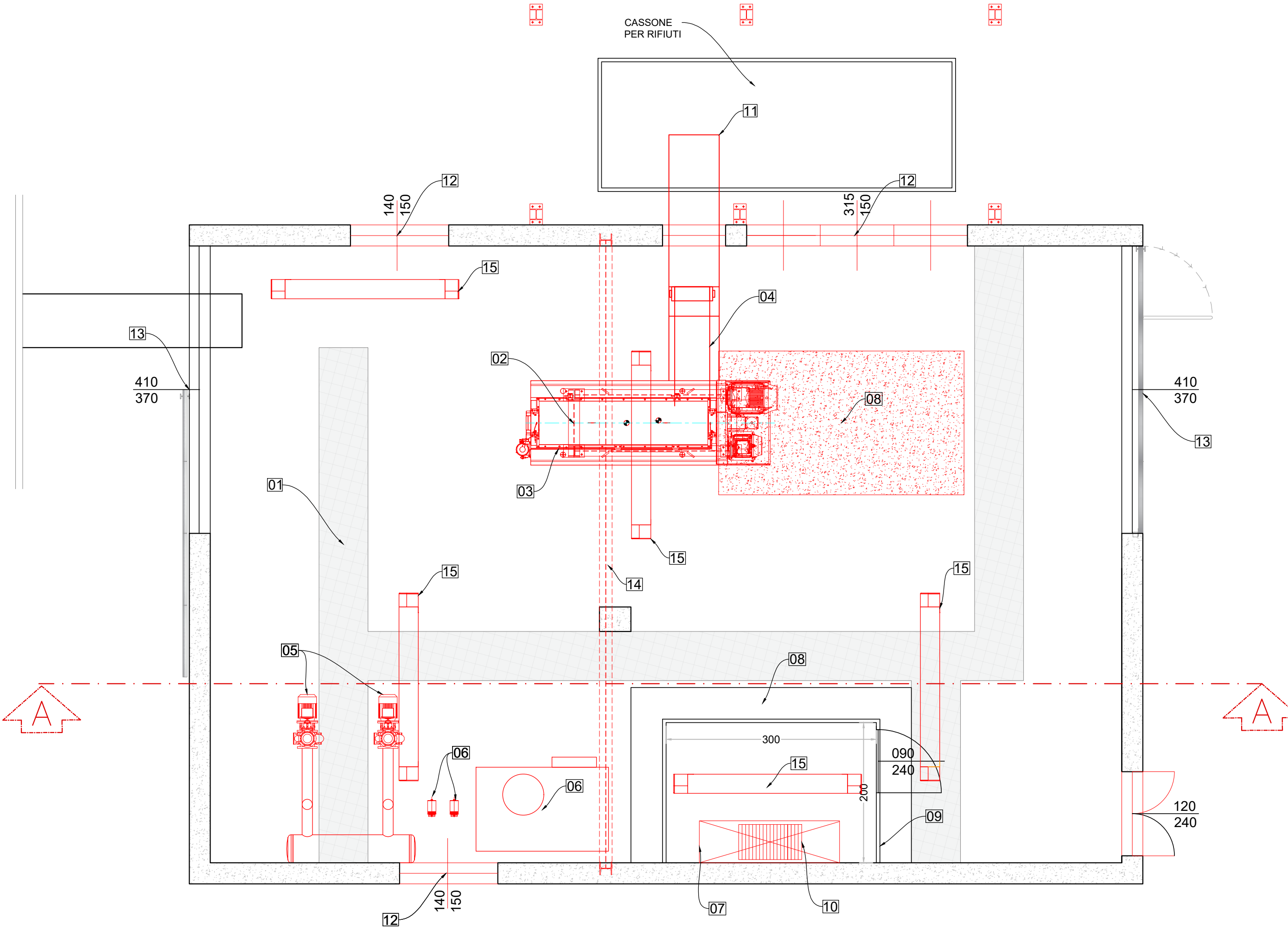
PIANTA LOCALE DISIDRATAZIONE FANGHI - OPERE IN PROGETTO SCALA - 1:50
