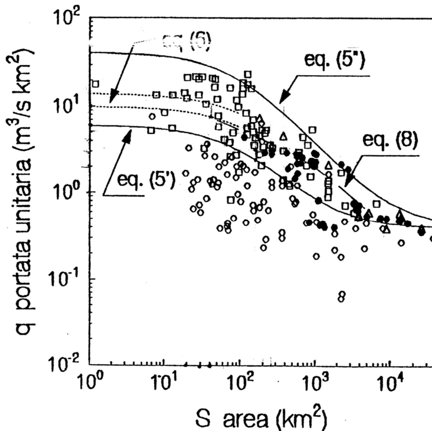
Figura 1 – Valori massimi delle portate al colmo osservate o indirettamente valutate in Piemonte, Valle d'Aosta e Ticino svizzero a fronte di alcune relazioni di involuppo dei valori con TR200 anni proposti dall'Autorità di Bacino per il Fiume Po (cerchi neri).
