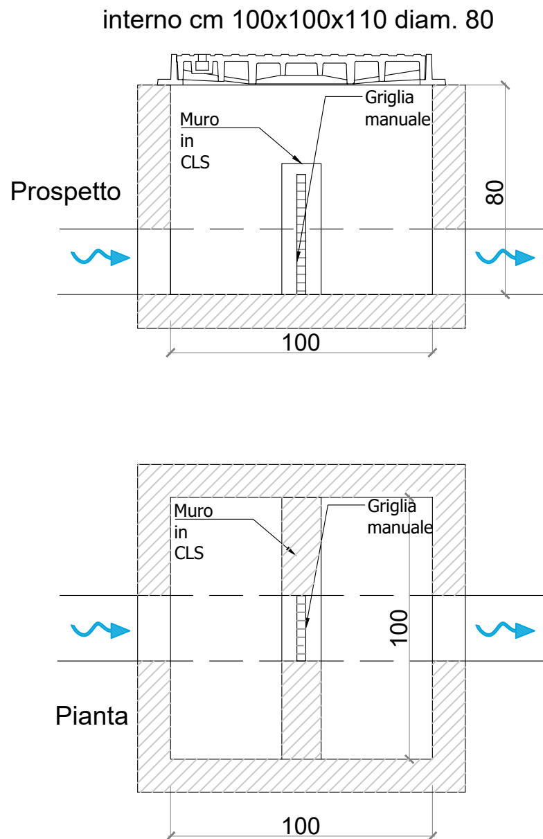
Pozzetto Griglia Manuale - Scala 1:20 -
