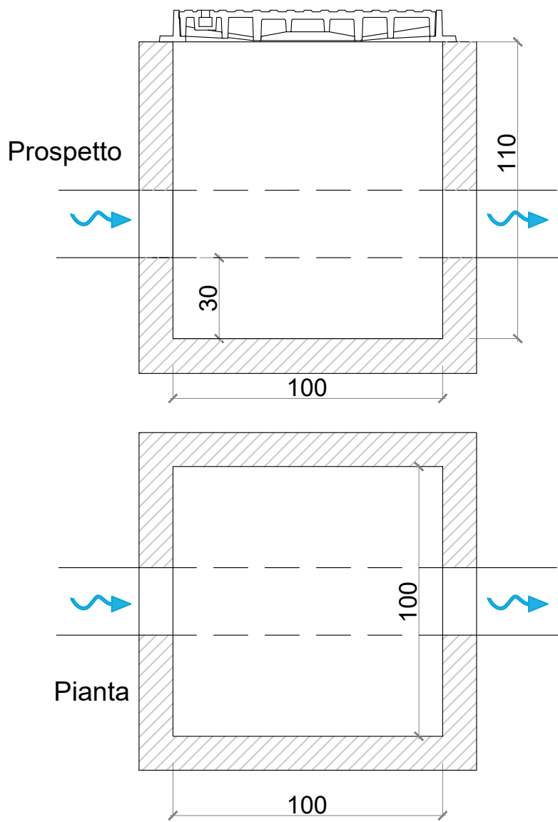
Pozzetto Prelievo Ingresso - Scala 1:20 -
