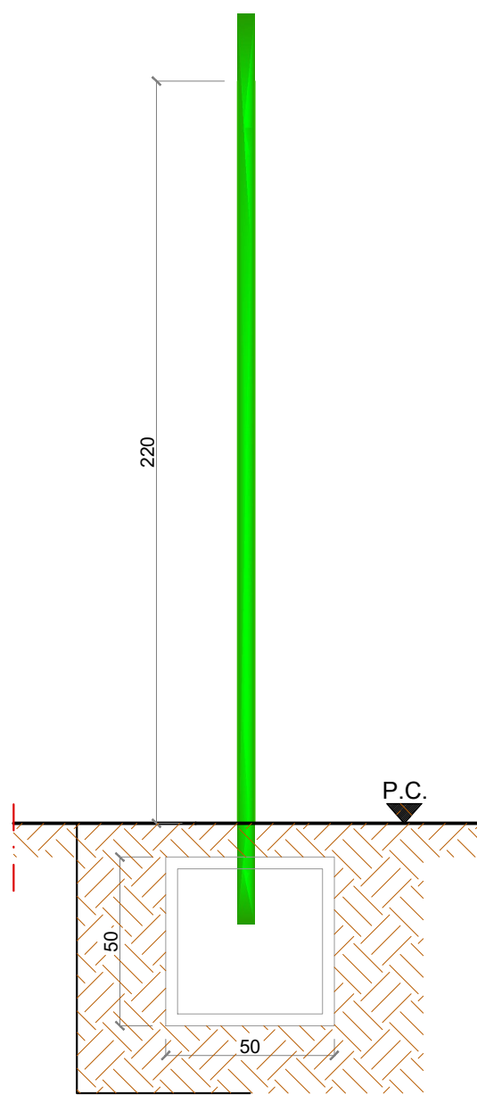
SEZIONE - Scala 1:20 -
