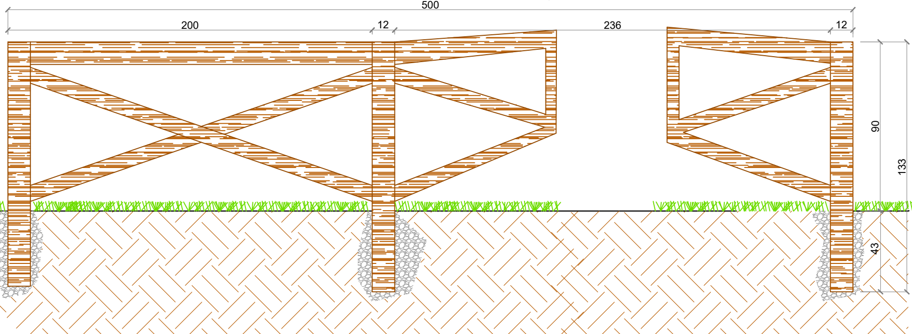
PARTICOLARE RECINZIONE (croce Sant'Andrea) Scala 1:20 Prospetti
