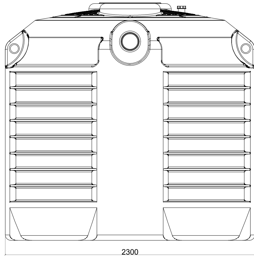
Imhoff corrugata 7000 norma UNI EN 12566-1 - Scala 1:200 -
