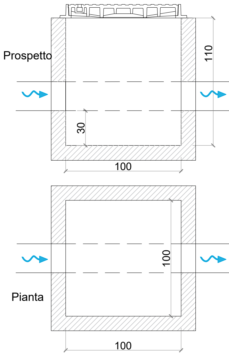
Pozzetto Prelievo Uscita / Compionamento - Scala 1:20 -
