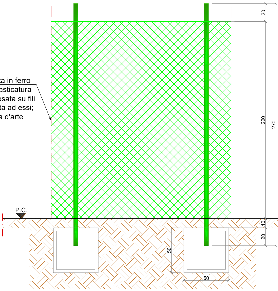
PROSPETTO - Scala 1:20 -
